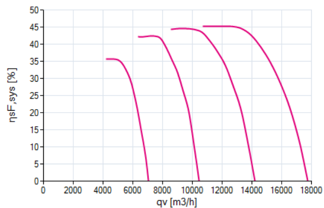
účinnost \eta_{sF,sys}
