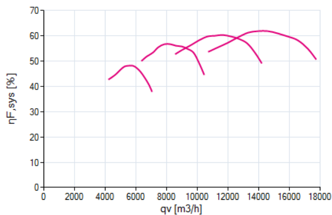
účinnost \eta_{F,sys}
