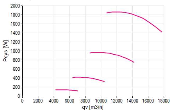
příkon P_{sys}
