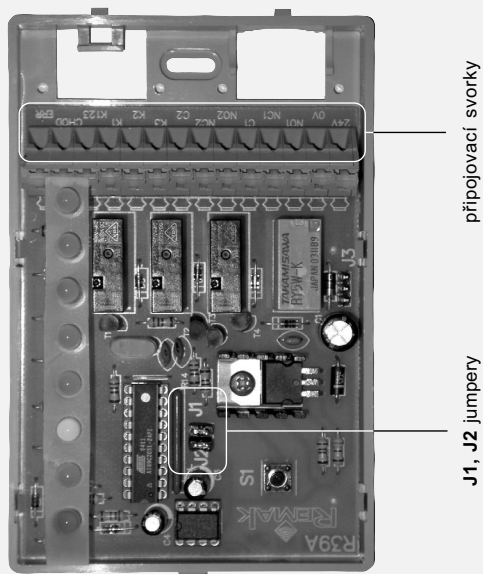
Obrázek 3 – připojení ovladače
