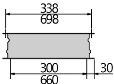
Seitenansicht
