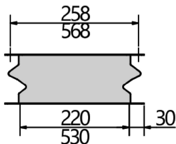
Seitenansicht
